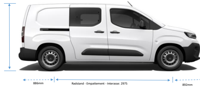
Berlingo Van Size XL Vertiefte Kabine / Cabine approfondie / Doppia Cabina
